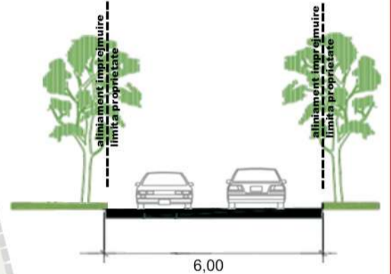
PROFIL ALEE CAROSABILA - propusa strada cat a IV-a - 2 benzi semicarosabil
